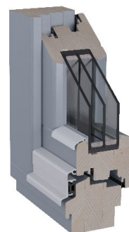
OKNO EURO DREWNO - „88 mm” U_w = 0.77 \text{ W/m}^2\text{K}
