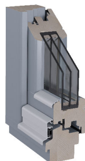
OKNO EURO DREWNO - „78 mm” U_w = 0.95 \text{ W/m}^2\text{K}
