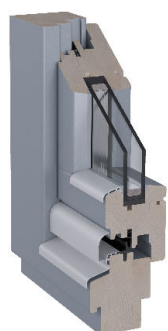
OKNO EURO DREWNO - „68 mm” U_w = 1.4 \text{ W/m}^2\text{K}
